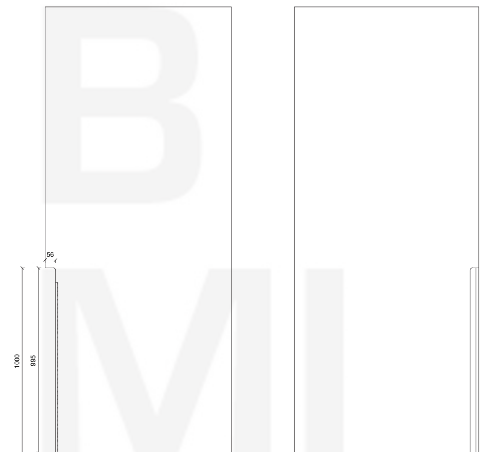
Aanzicht 1 deurblad met uitsnijding (zonder greep) - schaal 1/20
