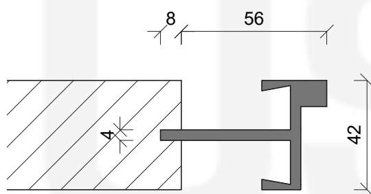
Doorsnede deurblad met greep - schaal 1/2
