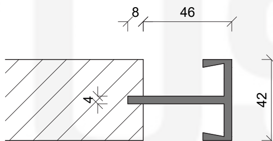
Doorsnede deurblad met greep - schaal 1/2
